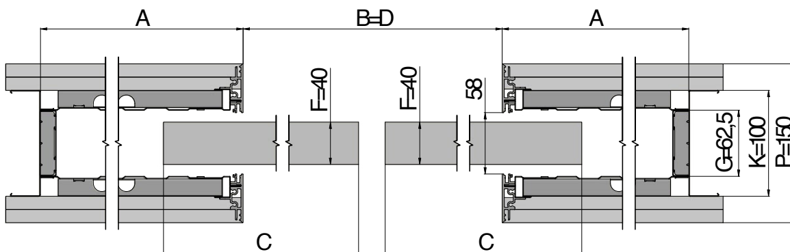
Horizontální řez pouzdem AKTIVE II KOMFORT dřevěným dveřním křídlem tloušťky 40 mm, tloušťka příčky 150 mm
