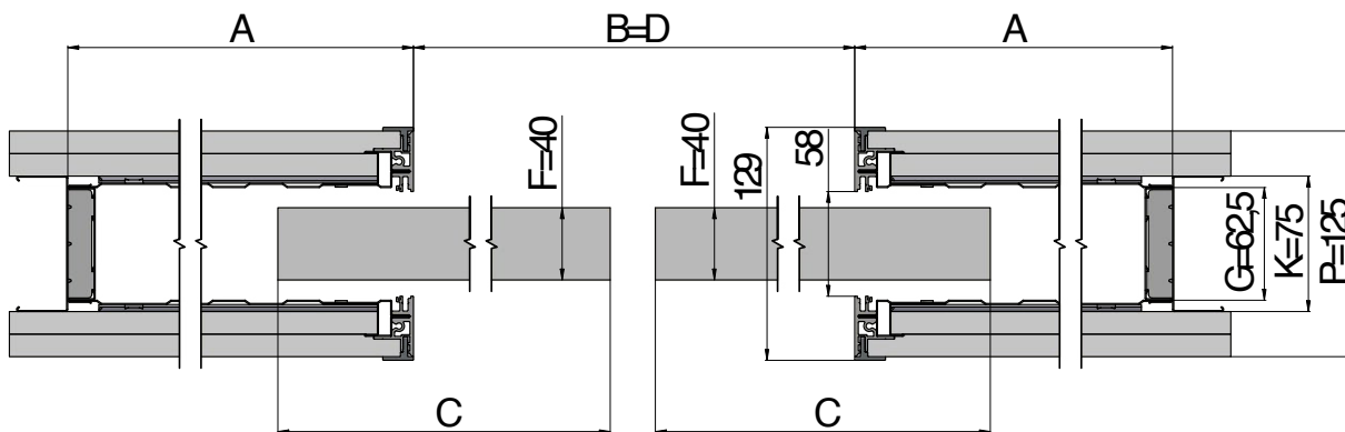
Horizontální řez pouzdrem EMOTIVEII KOMFORT dřevěným dveřním křídlem tloušťky 40 mm, tloušťka příčky 125 mm.
