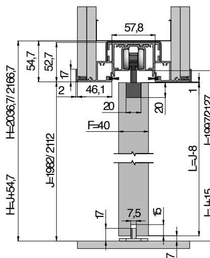
Vertikální řez pouzdrem EMOTIVEII KOMFORT dřevěným dveřním křídlem tloušťky 40 mm, tloušťka příčky 150 mm.
