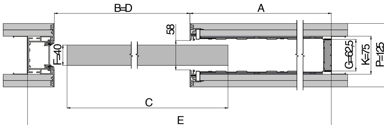
Horizontální řez pouzdem AKTIVE II STANDARD dřevěným dveřním křídlem tloušťky 40 mm, tloušťka příčky 125 mm.
