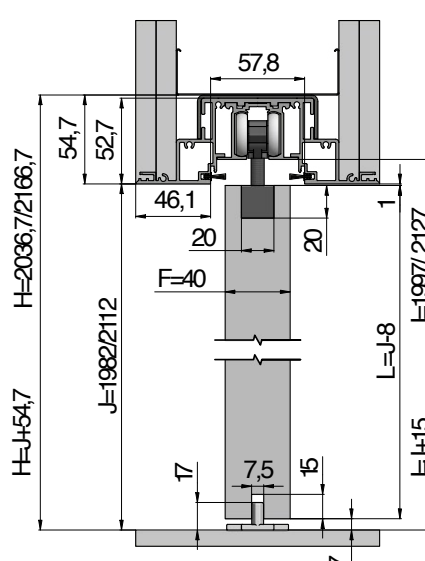
Vertikální řez pouzdem AKTIVE II KOMFORT dřevěným dveřním křídlem tloušťky 40 mm, tloušťka příčky 150 mm
