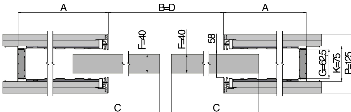
Horizontální řez pouzdem AKTIVE II KOMFORT dřevěným dveřním křídlem tloušťky 40 mm, tloušťka příčky 125 mm.
