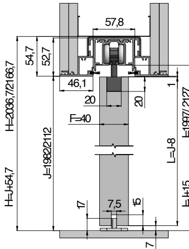
Vertikální řez pouzdem AKTIVE II STANDARD dřevěným dveřním křídlem tloušťky 40 mm, tloušťka příčky 150 mm.
