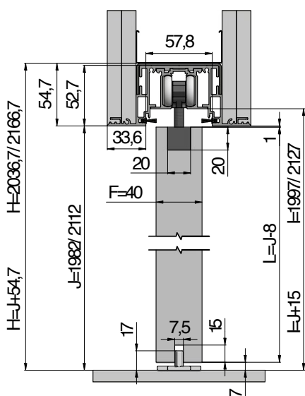
Vertikální řez pouzdem AKTIVE II KOMFORT dřevěným dveřním křídlem tloušťky 40 mm, tloušťka příčky 125 mm
