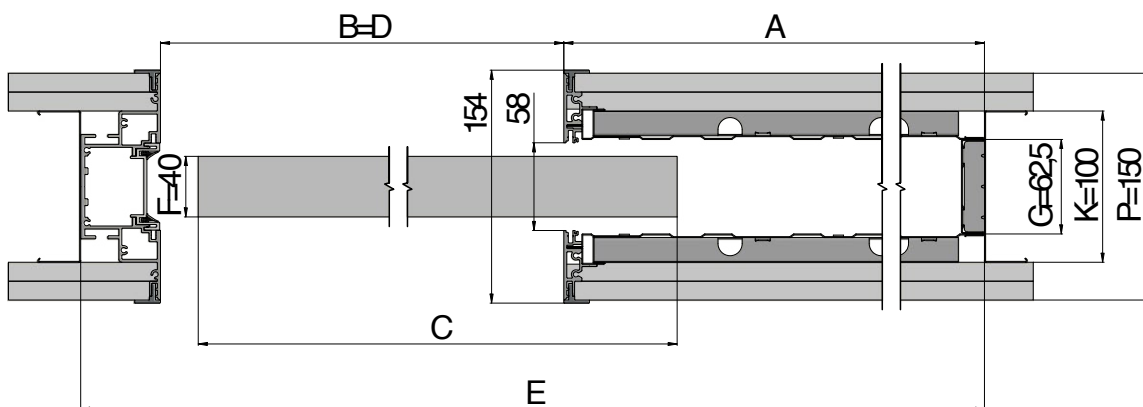
Horizontální řez pouzdrém EMOTIVE II STANDARD dřevěným dveřním křídlem tloušťky 40 mm, tloušťka příčky 150 mm.
