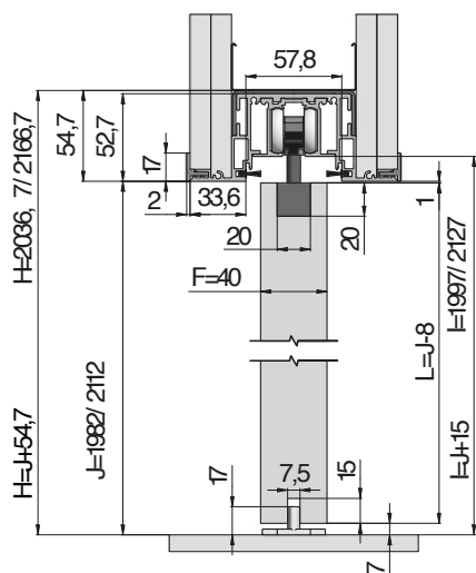
Vertikální řez pouzdrém EMOTIVE II STANDARD dřevěným dveřním křídlem tloušťky 40 mm, tloušťka příčky 125 mm.
