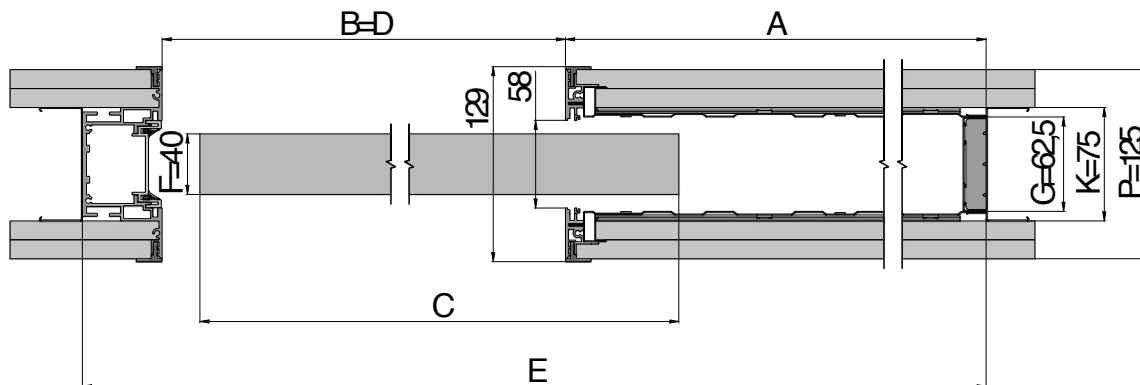
Horizontální řez pouzdrém EMOTIVE II STANDARD dřevěným dveřním křídlem tloušťky 40 mm, tloušťka příčky 125 mm.
