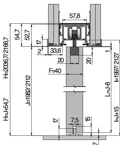
Vertikální řez pouzdrem EMOTIVEII KOMFORT dřevěným dveřním křídlem tloušťky 40 mm, tloušťka příčky 125 mm.
