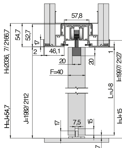
Vertikální řez pouzdrém EMOTIVE II STANDARD dřevěným dveřním křídlem tloušťky 40 mm, tloušťka příčky 150 mm.
