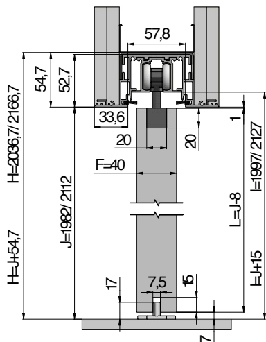
Vertikální řez pouzdem AKTIVE II STANDARD dřevěným dveřním křídlem tloušťky 40 mm, tloušťka příčky 125 mm.
