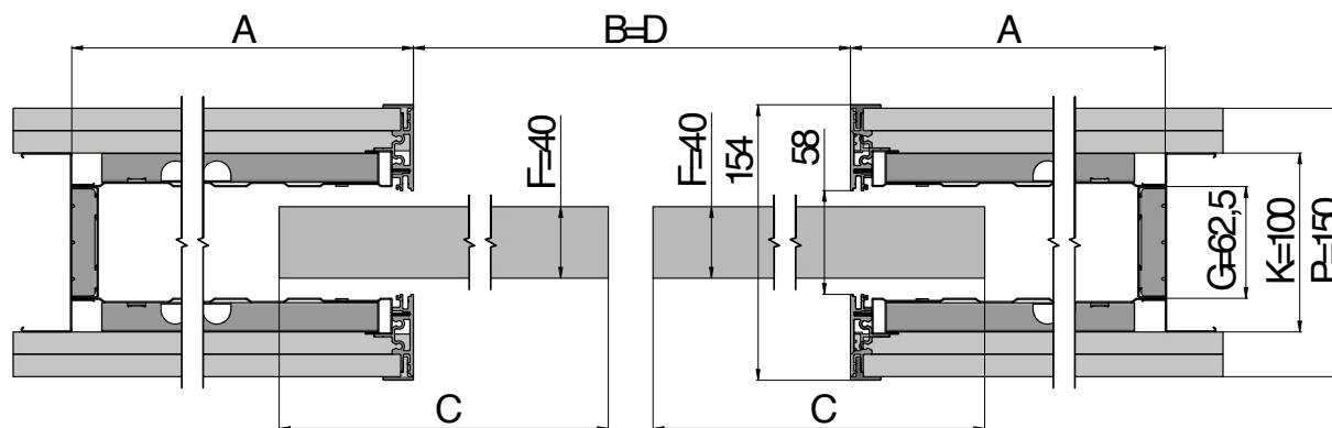
Horizontální řez pouzdrem EMOTIVEII KOMFORT dřevěným dveřním křídlem tloušťky 40 mm, tloušťka příčky 150 mm.
